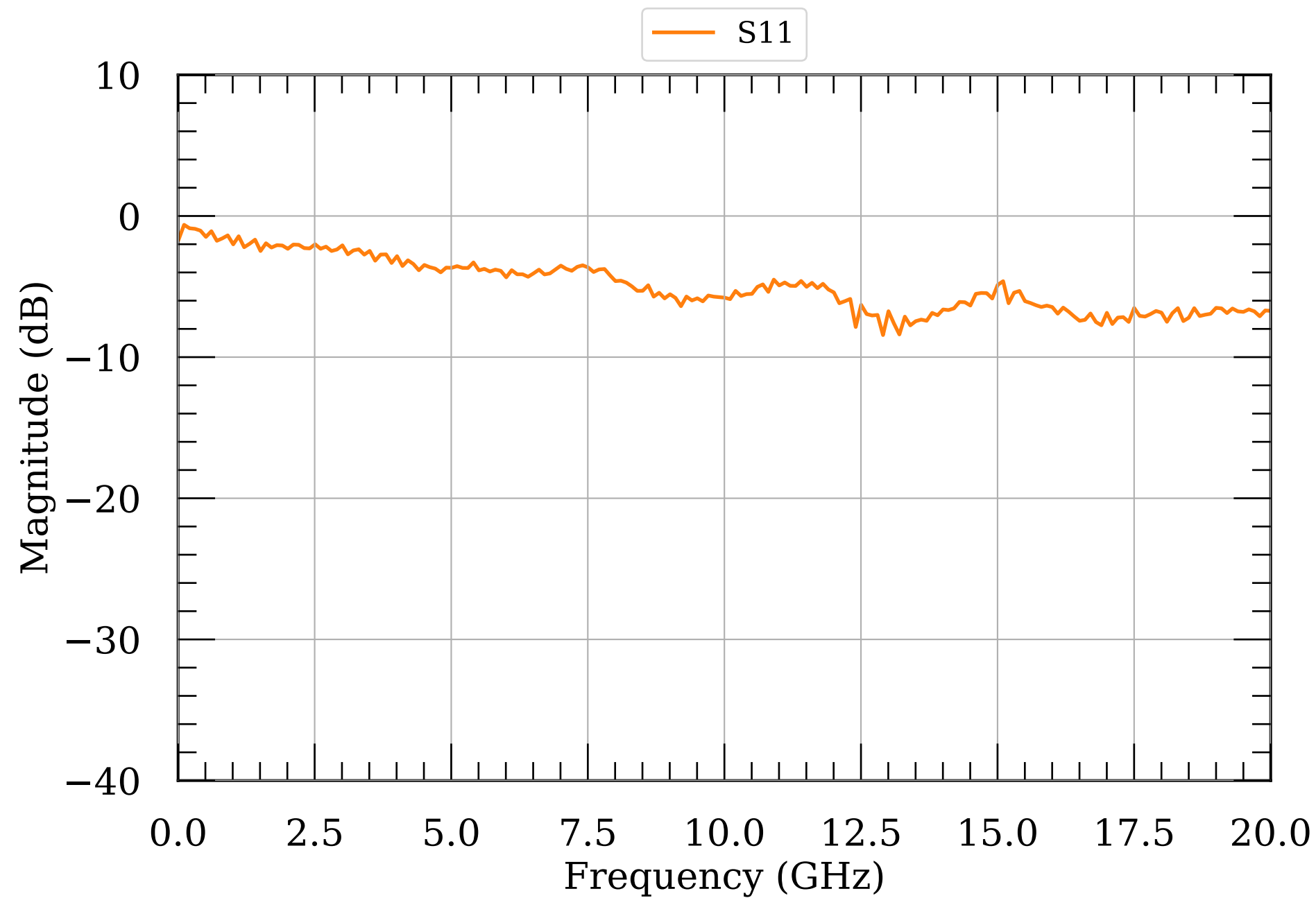
LNA S-params module020
